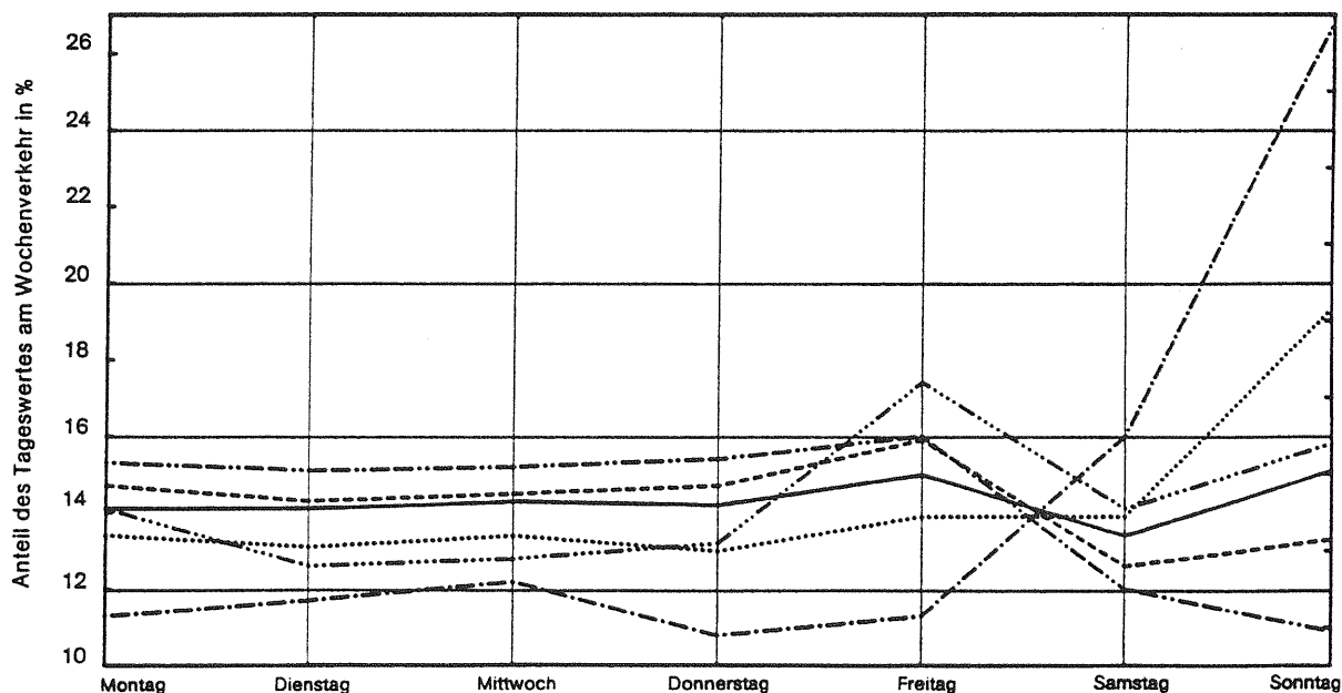
Bild 6: Jahresganglinientypen
