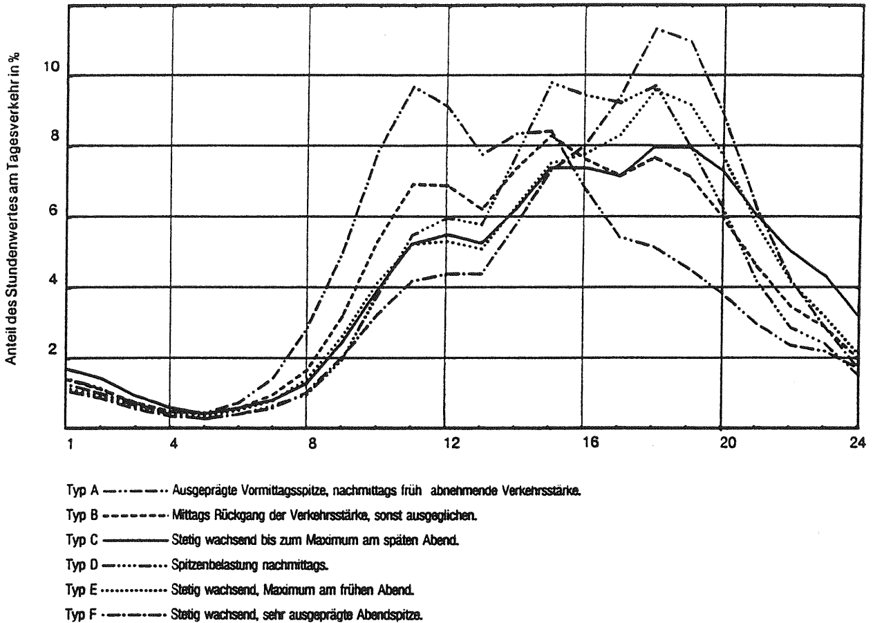
Bild 12: Tagesganglinien Sonntag
