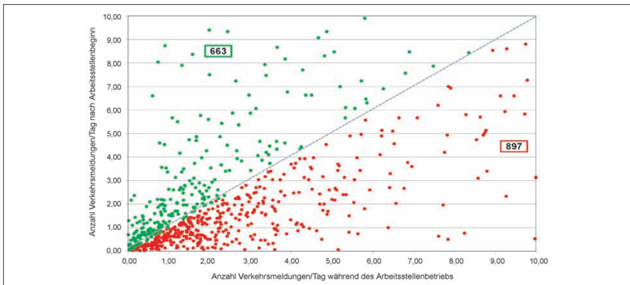
Bild 74: Gegenüberstellung der täglichen Verkehrsmeldungen während des Arbeitsstellenbetriebs und der täglichen Verkehrsmeldungen nach Arbeitsstellende für die Jahre 2006 und 2007
