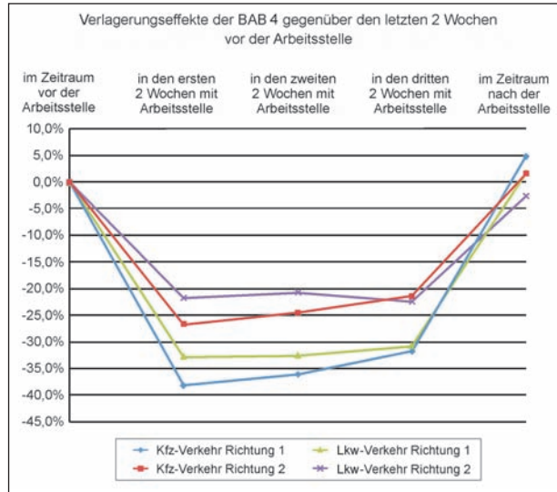
Bild 39: Veränderung der Verkehrsbelastungen bei Einrichtung der Arbeitsstelle auf der A 4 Bereich Wiehltal-Brücke
