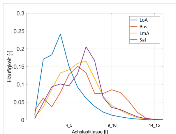
Bild 4-18: Repräsentative Achslastverteilungen der vier Schwerverkehrsklassen (alle AMS gleichgewichtet)
