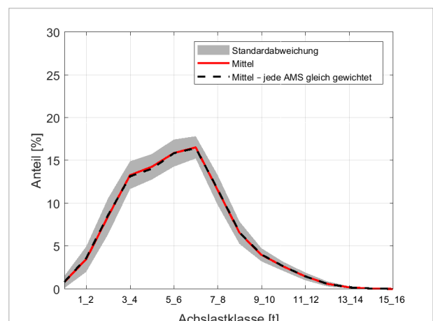
Bild 4-3: Repräsentative Achslastverteilung auf BAB - LmA
