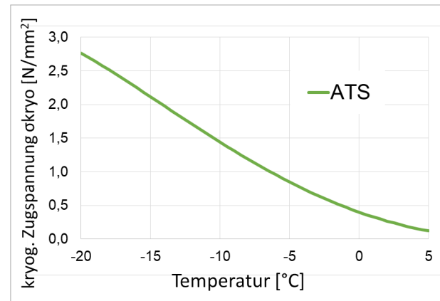
Bild 8-3: kryogene Zugspannungen des Kalibrierasphaltes der Asphalttragschicht
