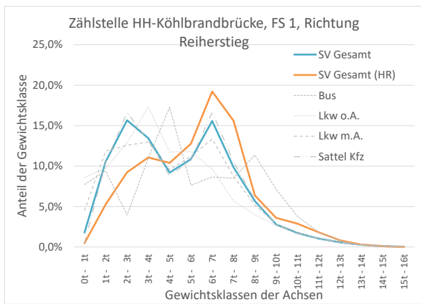
Bild 6-21: Vergleich Achslastverteilung real/HR Zst. Köhlbrandbrücke, FR Reierstieg, FS1
