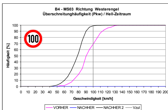
Bild 23: Überschreitungshäufigkeit an einem überwachten Messquerschnitt der B4
