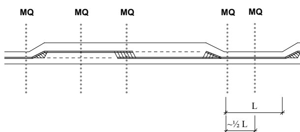
Bild 10: Messquerschnitte bei ÜFS mit kritischem Wechsel
