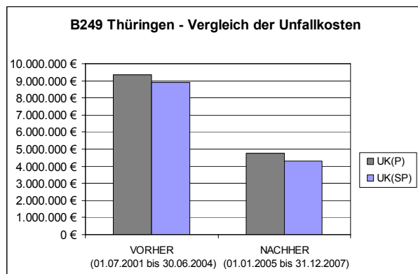
Bild 58: B249 Unfallkostenentwicklung
