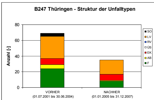
Bild 53: B247 Unfalltypenstruktur
