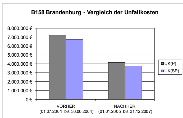
Bild 46: B158 Unfallkostenentwicklung
