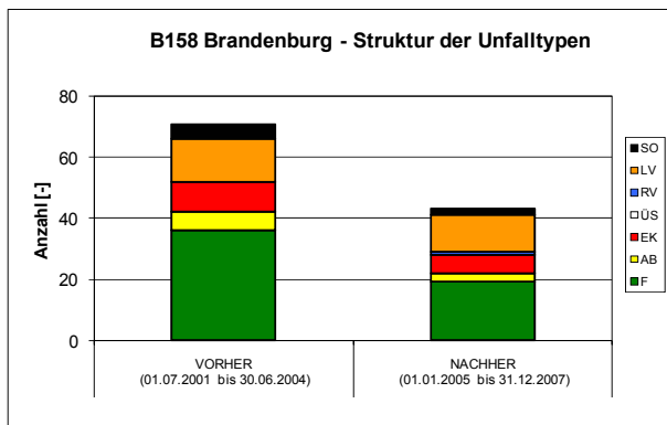
Bild 45: B158 Unfalltypenstruktur
