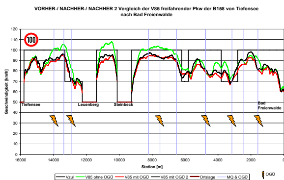
Bild 20: Geschwindigkeitsprofile B158 Richtung Bad Freienwalde
