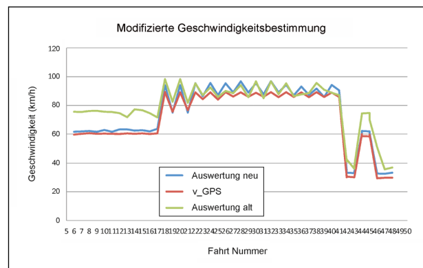
Bild 36: Ergebnisse der Geschwindigkeitsauswertung mit modifizierten Parametern
