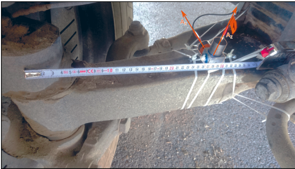
Bild 10: Beschleunigungssensoren auf der rechten Vorderachse
