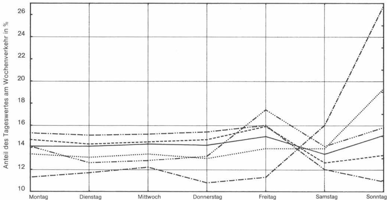
Bild 3: Jahresganglinientypen
