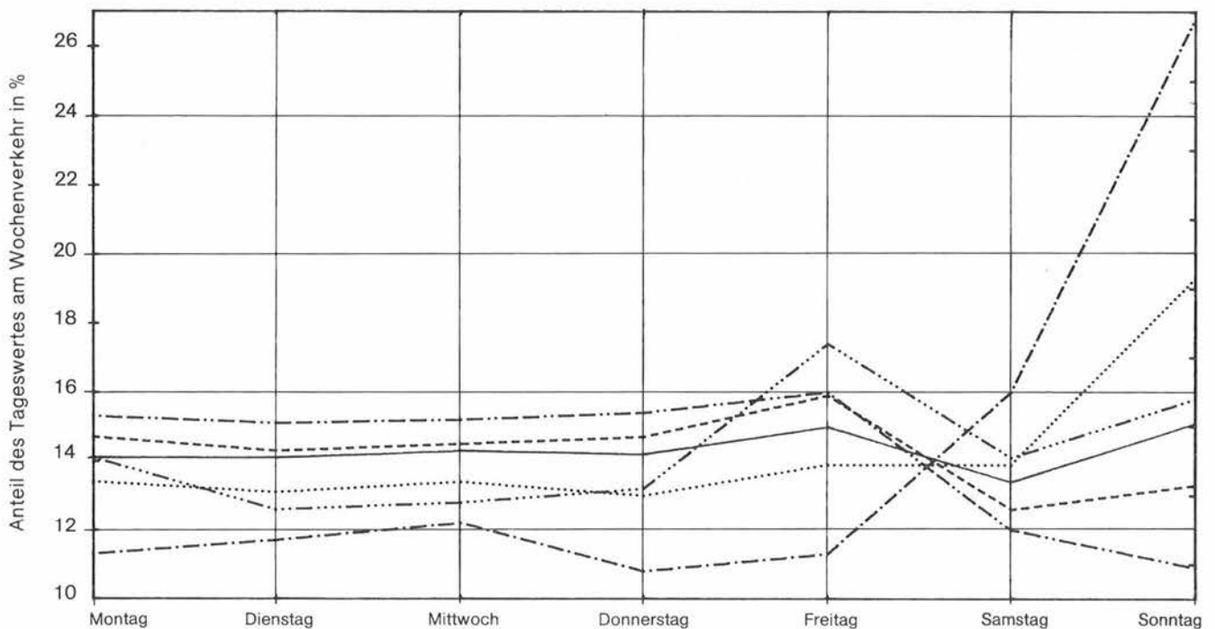
Bild 6: Jahresganglinientypen
