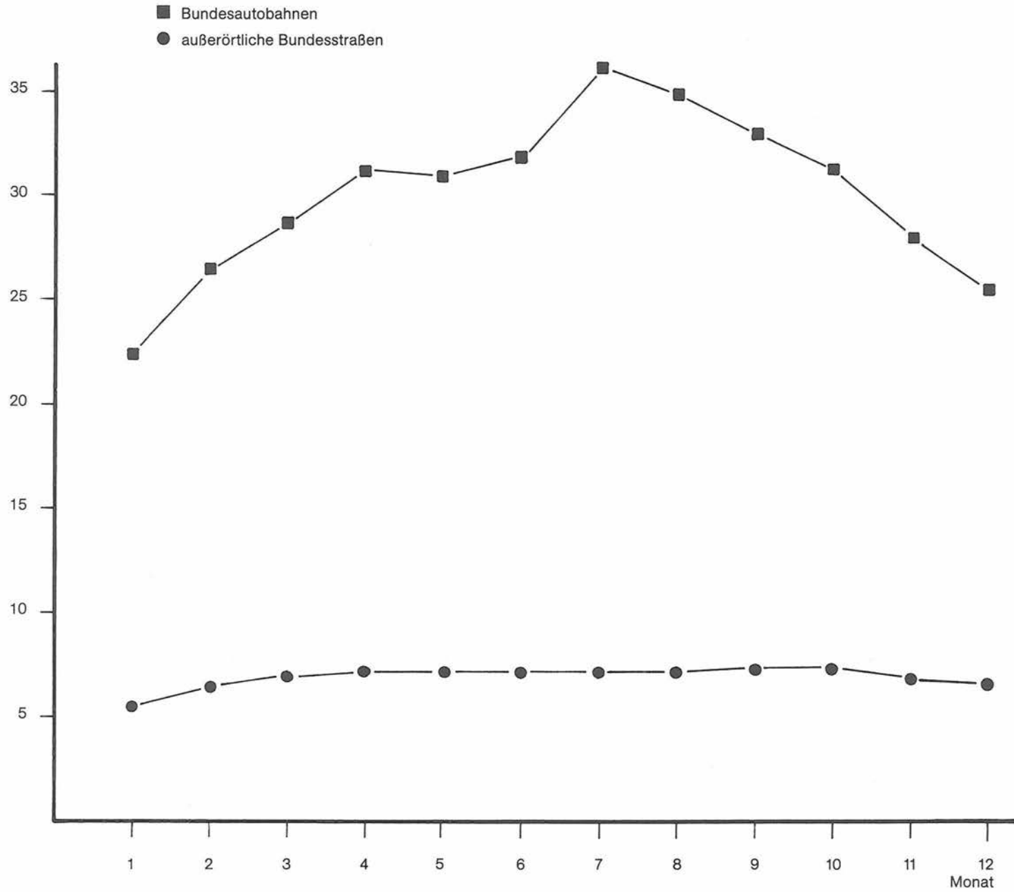
Bild 5: Mittlere DTV-Werte 1982 für Bundesautobahnen und außerörtliche Bundesstraßen
