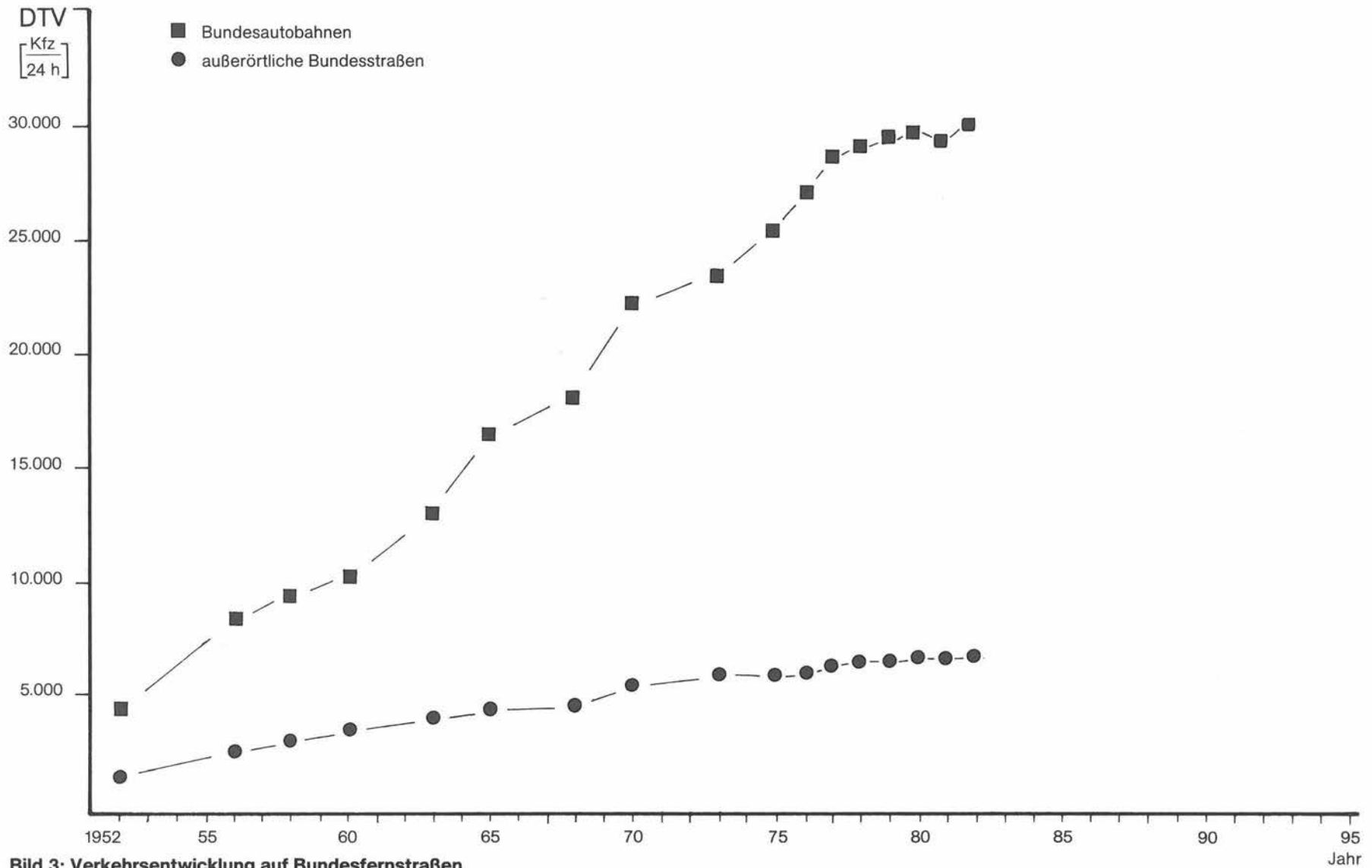
Bild 3: Verkehrsentwicklung auf Bundesfernstraßen
