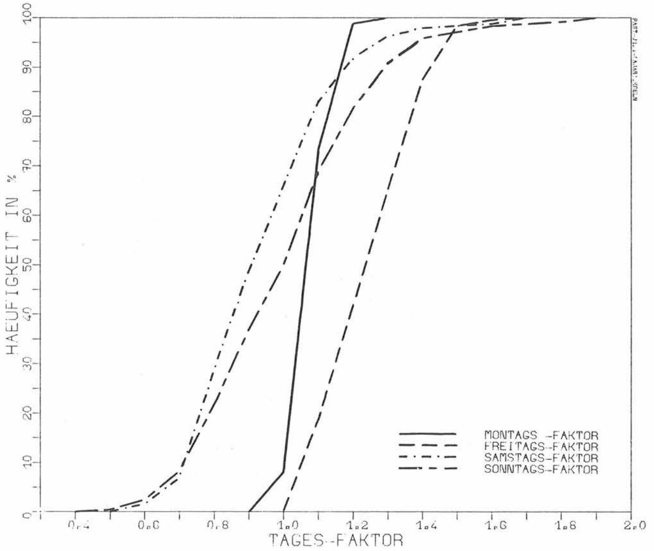
Bild 12: Verteilung der querschnittsbezogenen Wochentagsfaktoren der Zählstellen auf Bundesautobahnen
