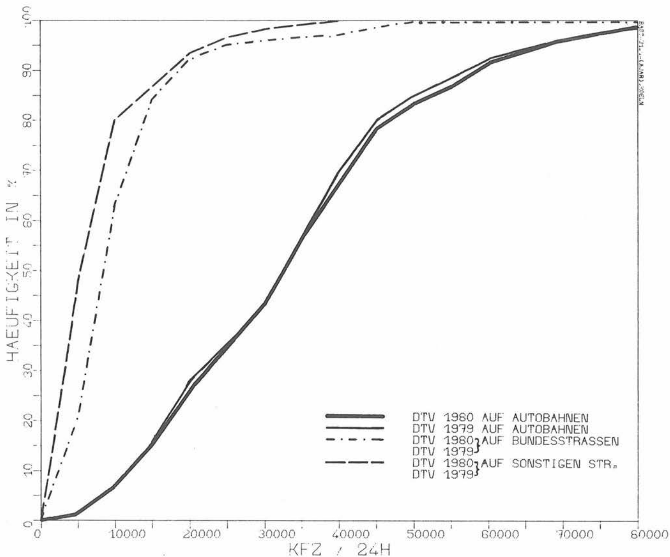
Bild 7: Verteilungsfunktion der DTV-Werte an Langzeitzählstellen 1979 und 1980
