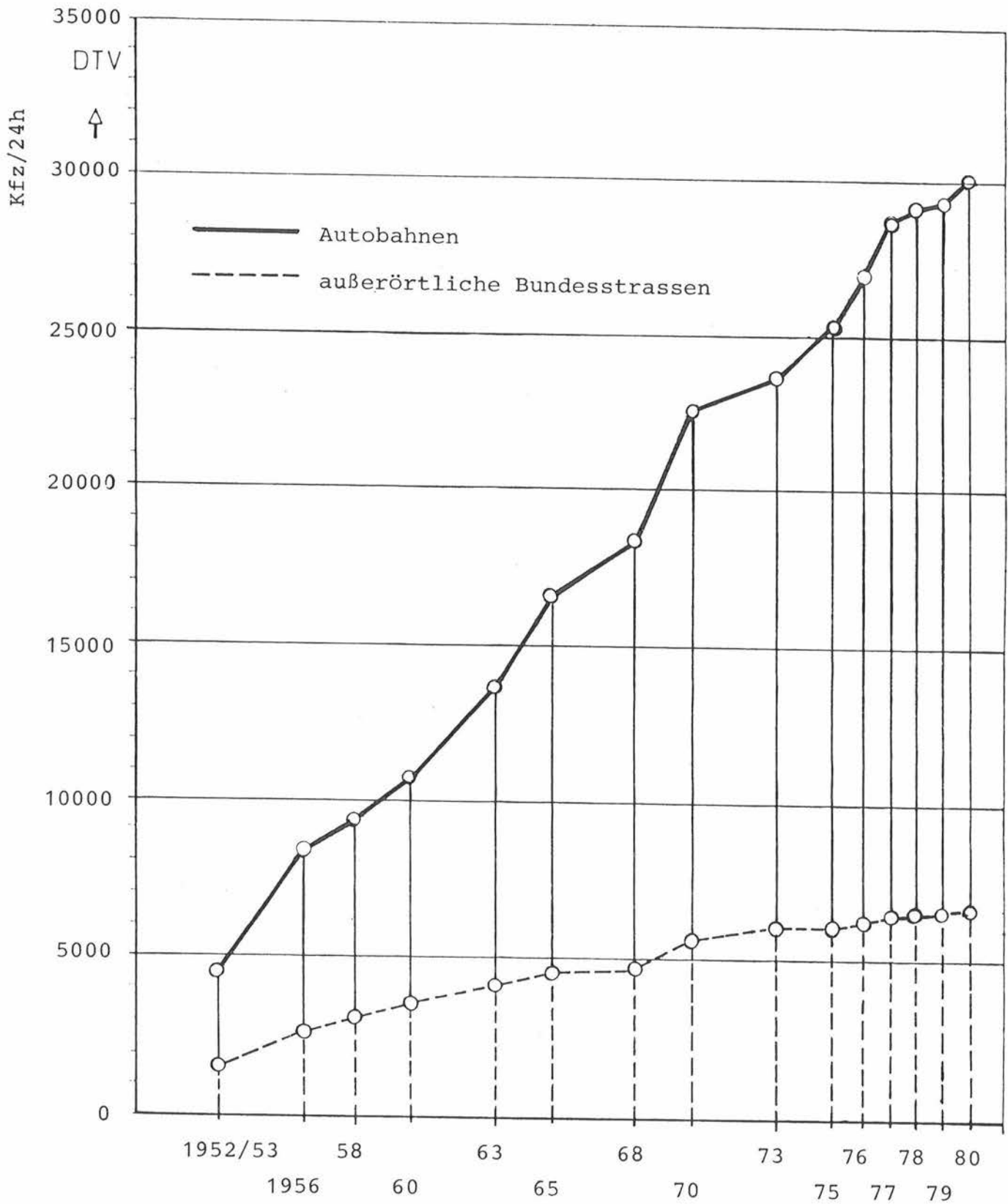
Bild 9: Verkehrsentwicklung auf Bundesstraßen
