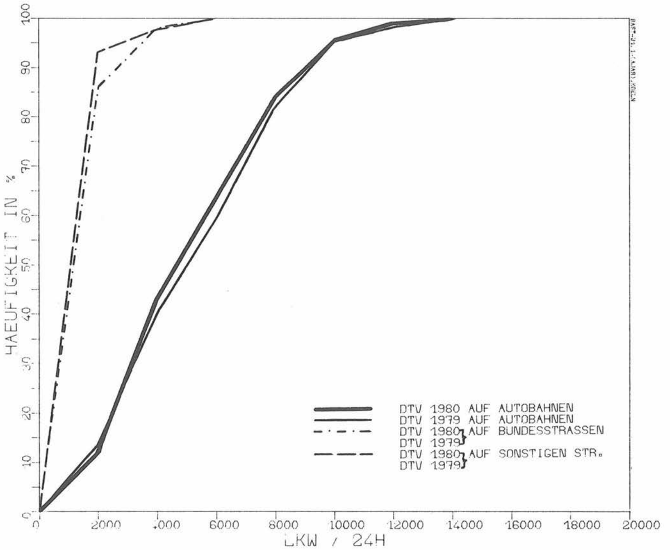
Bild 11: Verteilungsfunktion der DTV L -WERTE an Langzeitzählstellen 1979 L und 1980
