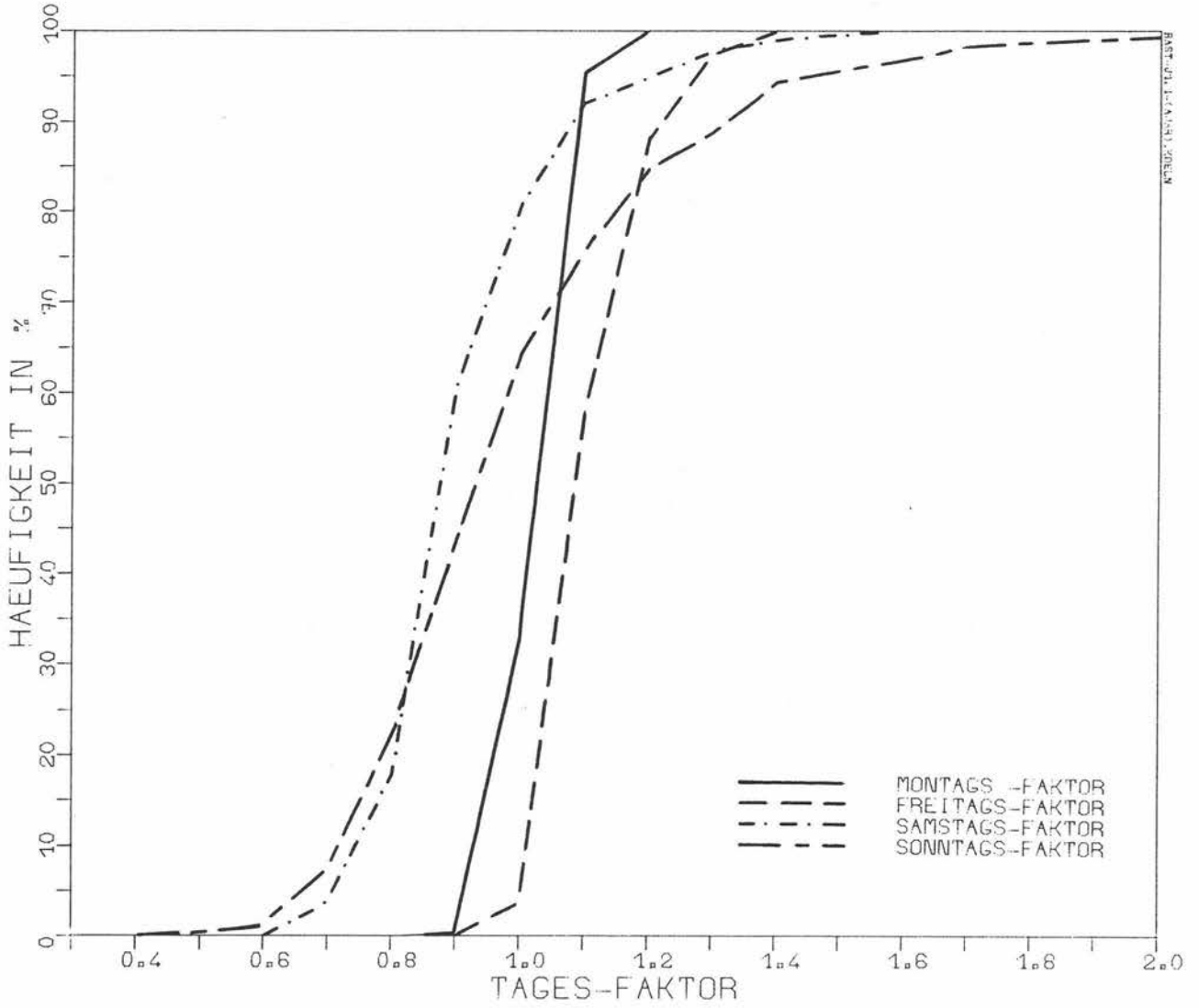
Bild 13: Verteilung der querschnittsbezogenen Wochentagsfaktoren der Zählstellen auf Bundesstraßen
