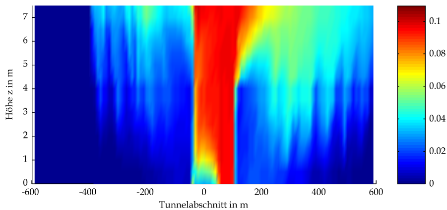
BAStBÜ Gewölbe Mulde GV 300 CO 2 -Gehalt in Masse-% bei t=180s
