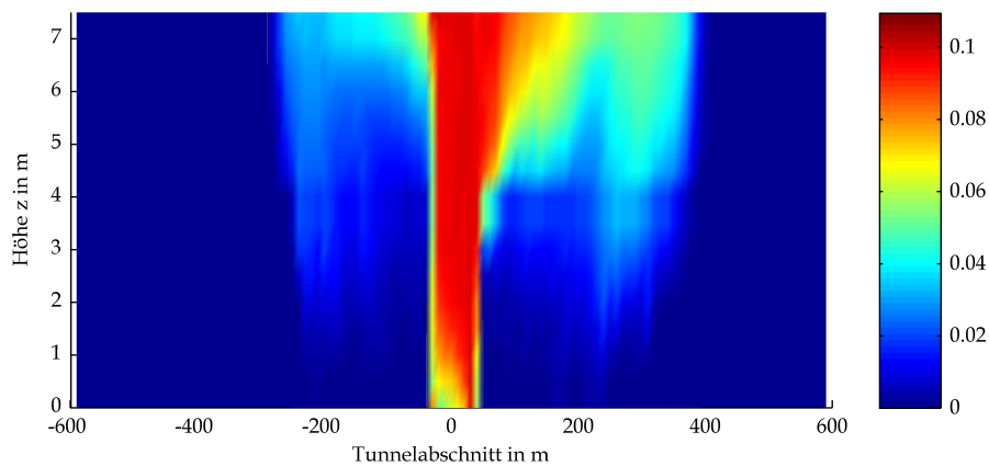
BAStBÜ Gewölbe Mulde GV 300 CO 2 -Gehalt in Masse-% bei t=120s
