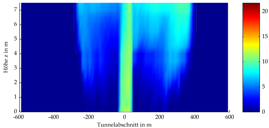
BAStBÜ Gewölbe Mulde GV 300 Optische Dichte bei t=120s
