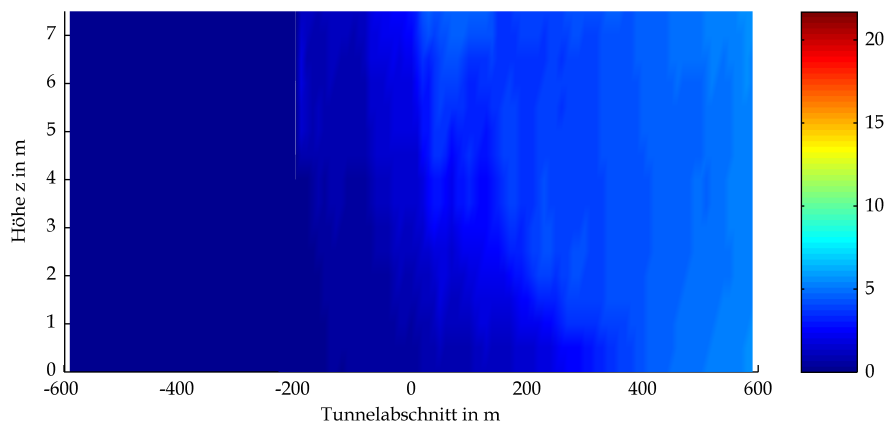
BAStBÜ Gewölbe Mulde GV 300 Optische Dichte bei t=2400s
