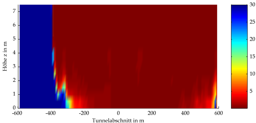
BASTBÜ Gewölbe Mulde GV 300 Sichtbarkeit in m bei t=180s
