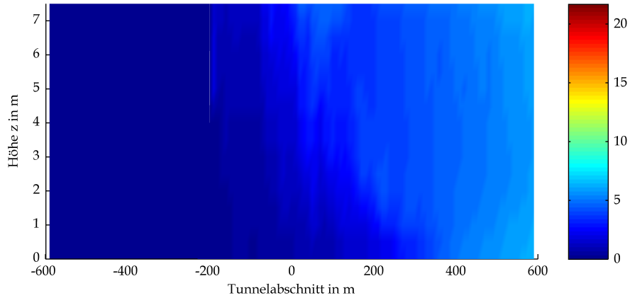
BAStBÜ Gewölbe Mulde GV 300 Optische Dichte bei t=1200s
