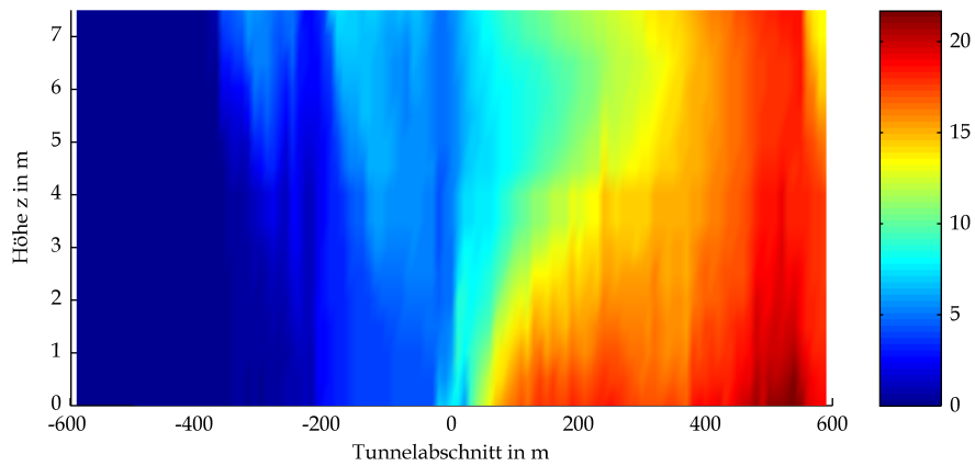
BAStBÜ Gewölbe Mulde GV 300 Optische Dichte bei t=600s
