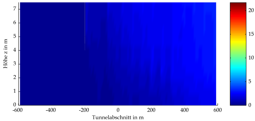
BAStBÜ Gewölbe Mulde GV 300 Optische Dichte bei t=3900s
