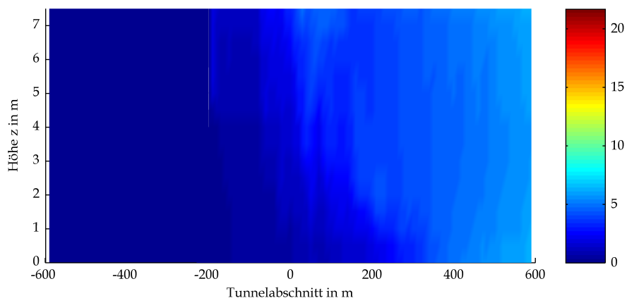
BAStBÜ Gewölbe Mulde GV 300 Optische Dichte bei t=1500s
