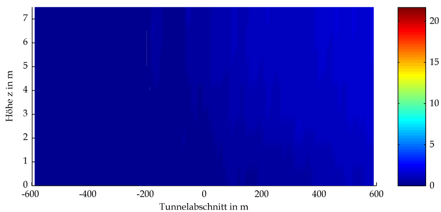
BAStBÜ Gewölbe Mulde GV 300 Optische Dichte bei t=4200s
