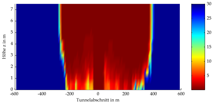
BASTBÜ Gewölbe Mulde GV 300 Sichtbarkeit in m bei t=120s
