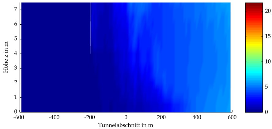
BAStBÜ Gewölbe Mulde GV 300 Optische Dichte bei t=2100s
