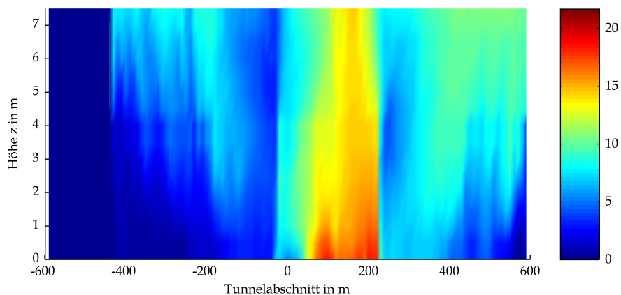
BAStBÜ Gewölbe Mulde GV 300 Optische Dichte bei t=180s
