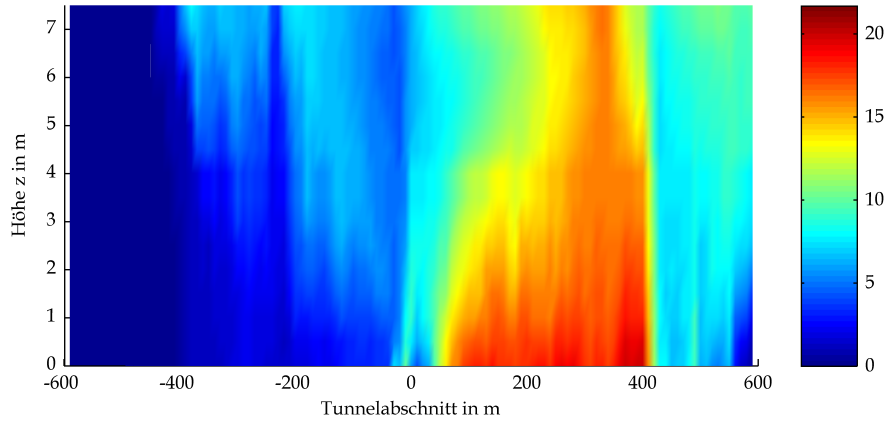
BAStBÜ Gewölbe Mulde GV 300 Optische Dichte bei t=300s
