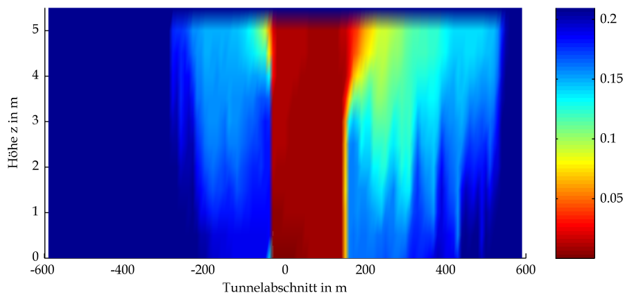
BAStBÜ Rechteck Mulde GV 300 owF Sauerstoffkonzentration in Vol-% bei t=180s
