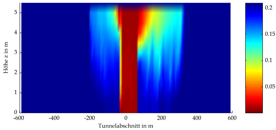
BAStBÜ Rechteck Mulde GV 300 owF Sauerstoffkonzentration in Vol-% bei t=120s
