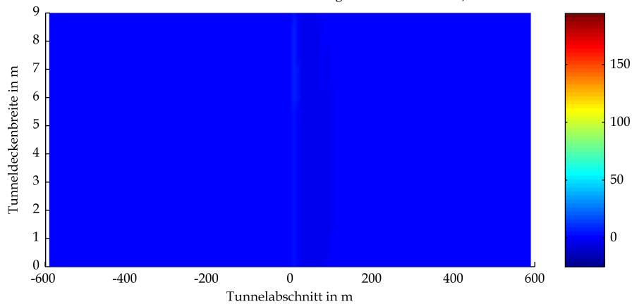
BAStBÜ Rechteck Mulde GV 300 owF Wärmestrahlung Tunneldecke in kW/m 2 bei t=3300s
