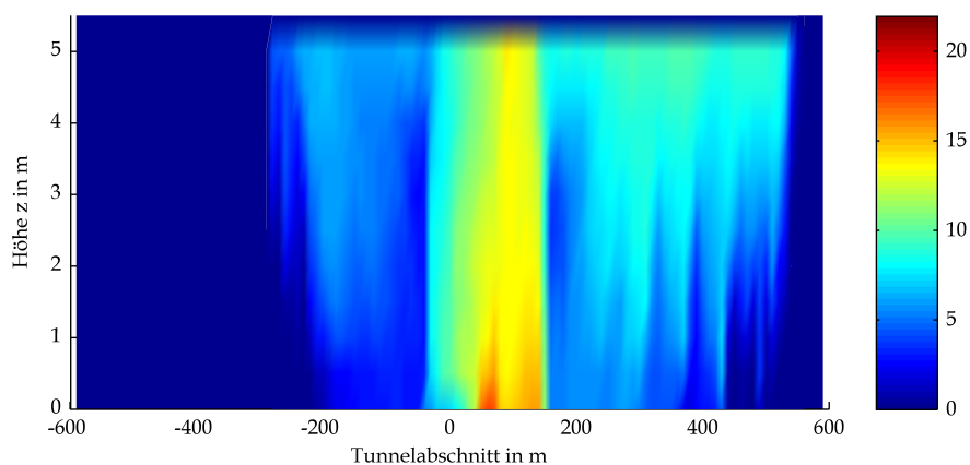
BASStBÜ Rechteck Mulde GV 300 owF Optische Dichte bei t=180s
