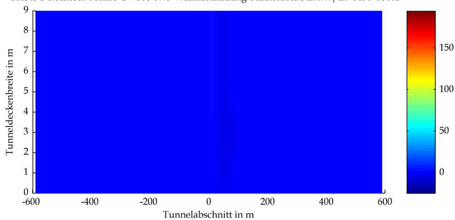
BAStBÜ Rechteck Mulde GV 300 owF Wärmestrahlung Tunneldecke in kW/m 2 bei t=3300s
