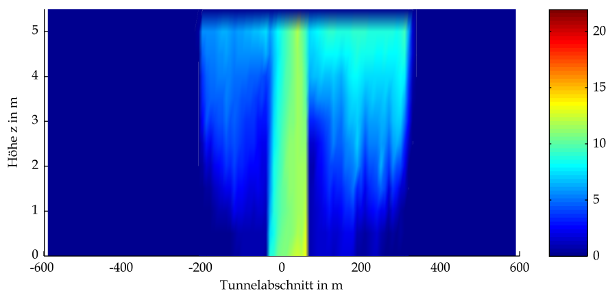
BASStBÜ Rechteck Mulde GV 300 owF Optische Dichte bei t=120s
