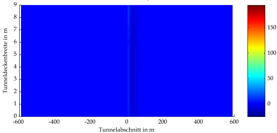
BAStBÜ Rechteck Mulde GV 300 owF Wärmestrahlung Tunneldecke in kW/m 2 bei t=2400s
