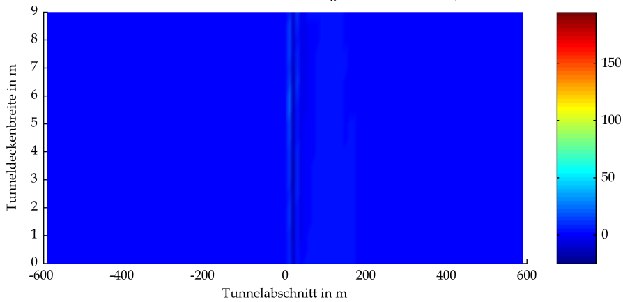
BAStBÜ Rechteck Mulde GV 300 owF Wärmestrahlung Tunneldecke in kW/m 2 bei t=2100s
