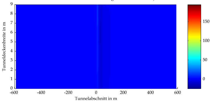
BAStBÜ Rechteck Mulde GV 300 owF Wärmestrahlung Tunneldecke in kW/m 2 bei t=2400s
