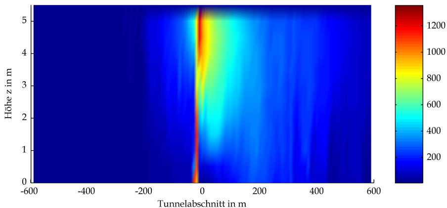
BAStBÜ Rechteck Mulde GV 300 owF Gastemperaturen in °C bei t=180s
