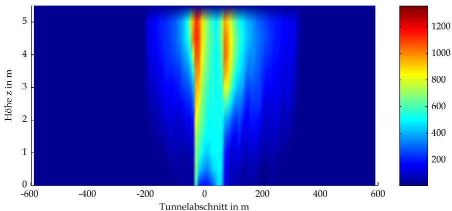
BAStBÜ Rechteck Mulde GV 300 owF Gastemperaturen in °C bei t=120s
