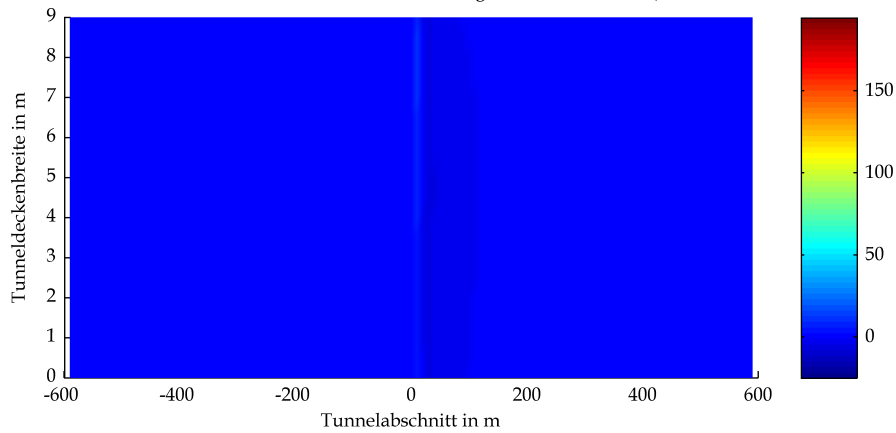
BAStBÜ Rechteck Mulde GV 300 owF Wärmestrahlung Tunneldecke in kW/m 2 bei t=3000s
