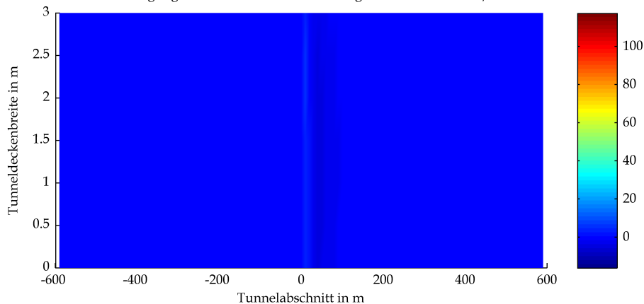
BAStBÜ Gewölbe Neigung GV 20.6 owF Wärmestrahlung Tunneldecke in kW/m 2 bei t=2400s
