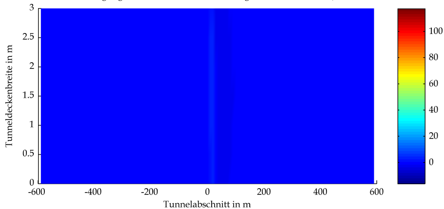
BAStBÜ Gewölbe Neigung GV 20.6 owF Wärmestrahlung Tunneldecke in kW/m 2 bei t=3000s
