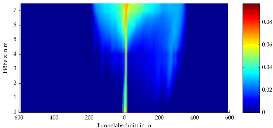
BAStBÜ Gewölbe Neigung GV 20.6 owF CO 2 -Gehalt in Masse-% bei t=120s
