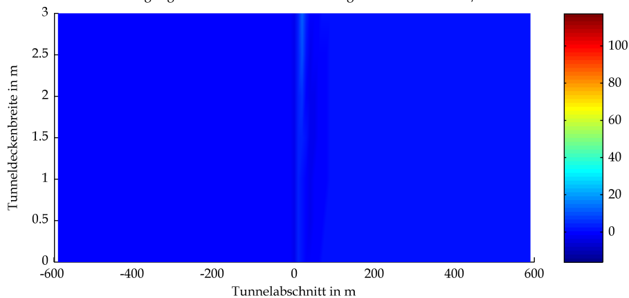
BAStBÜ Gewölbe Neigung GV 20.6 owF Wärmestrahlung Tunneldecke in kW/m 2 bei t=2100s
