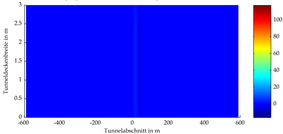
BAStBÜ Gewölbe Neigung GV 20.6 owF Wärmestrahlung Tunneldecke in kW/m 2 bei t=3300s
