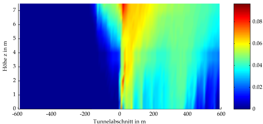
BAStBÜ Gewölbe Neigung GV 20.6 owF CO 2 -Gehalt in Masse-% bei t=180s
